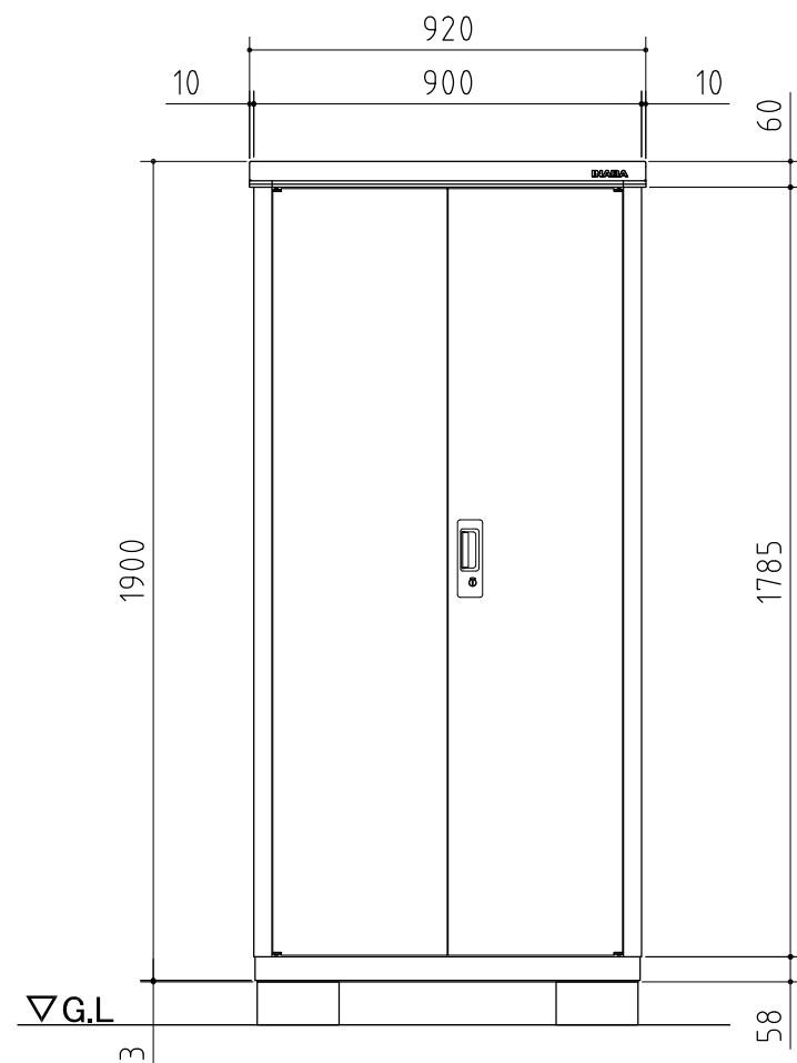
正面図
