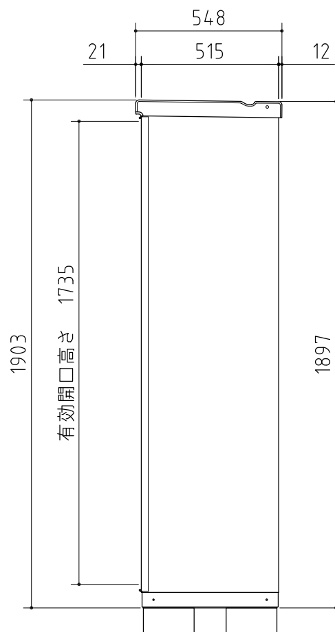
側面図
