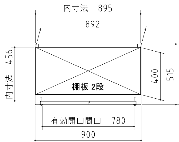
平面図
