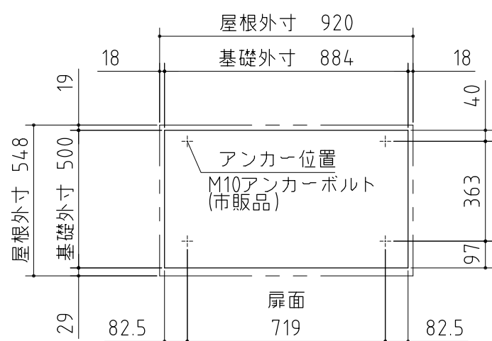
ベタ基礎図
